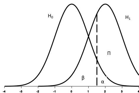
Figuur 1: Overzicht type I/II fouten en power
